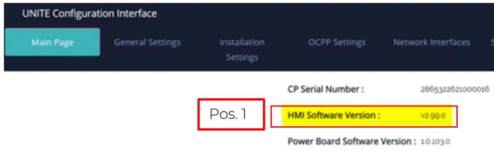
Abbildung 2-1: Softwareversion
