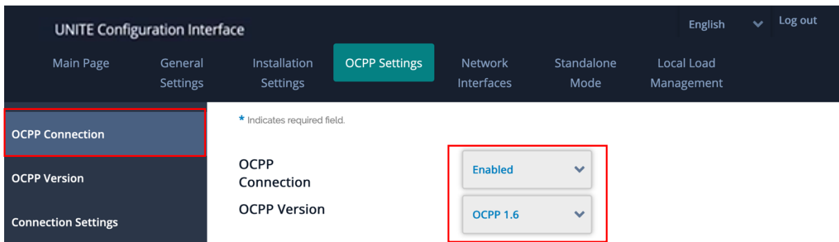
Abbildung 2-2: OCPP-Auswahl
