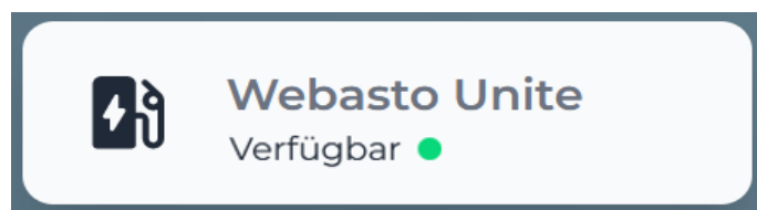
Abbildung 2-5: Anbindungsstatus
